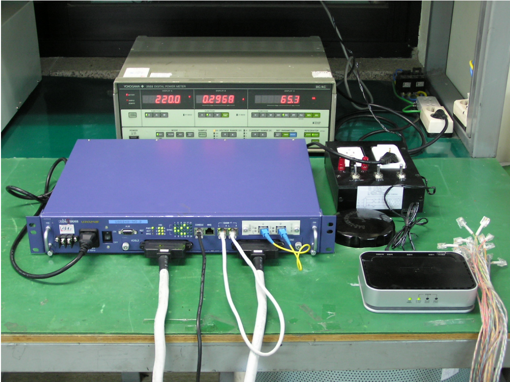
누설전류 시험
