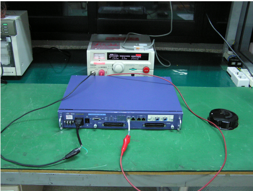
누설전류 시험
