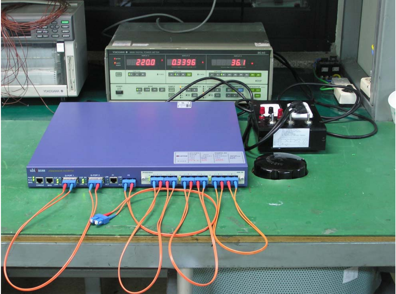
소비전력 시험
