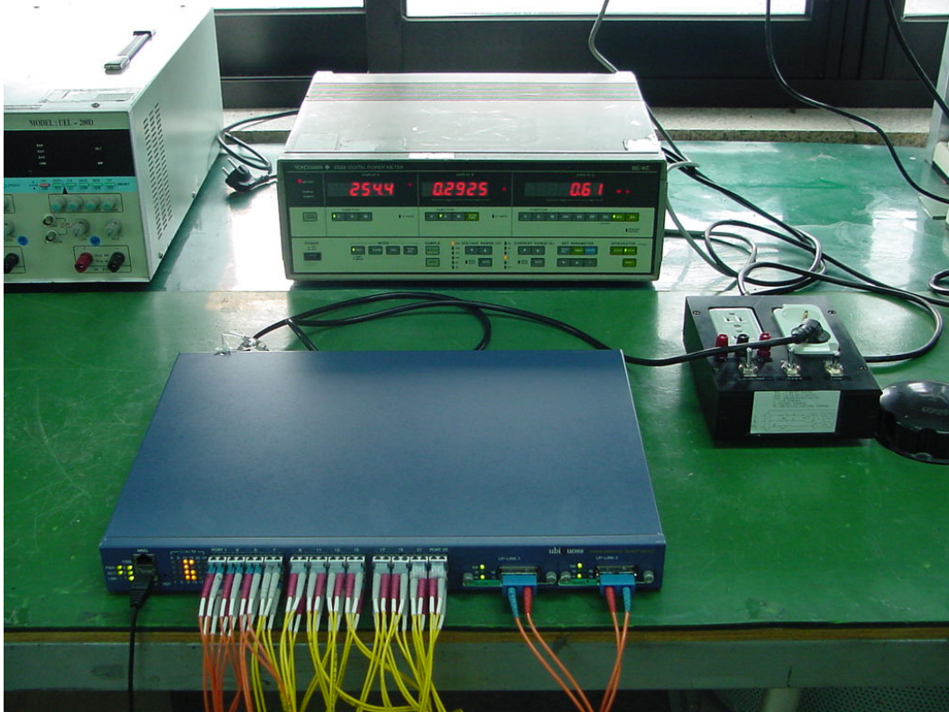
누설전류 시험
