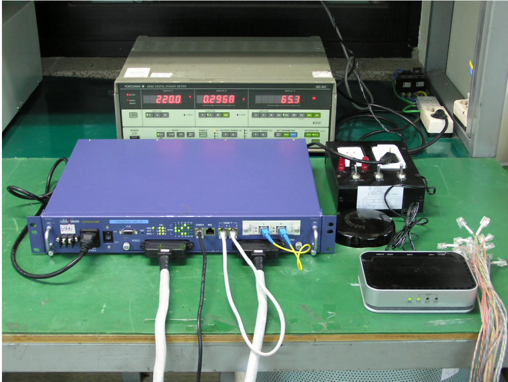
누설전류 시험
