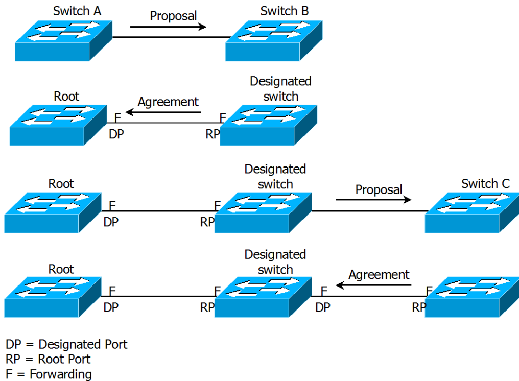
그림 8-3. Proposal and Agreement Handshaking for Rapid Convergence
