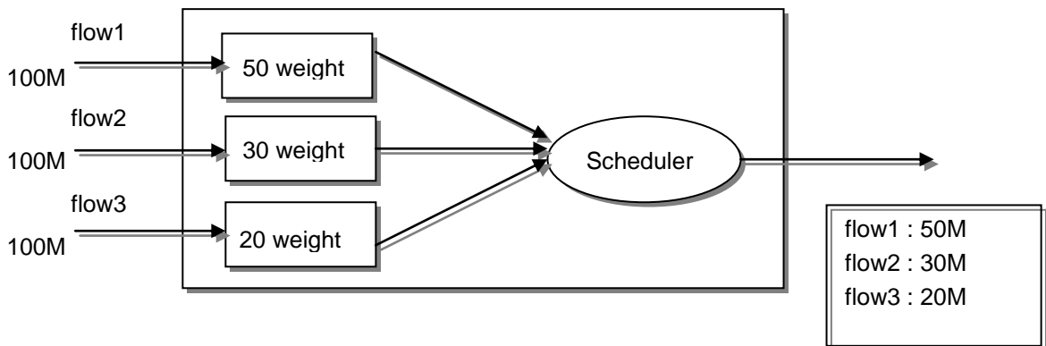
그림 10-3. WRR Method
