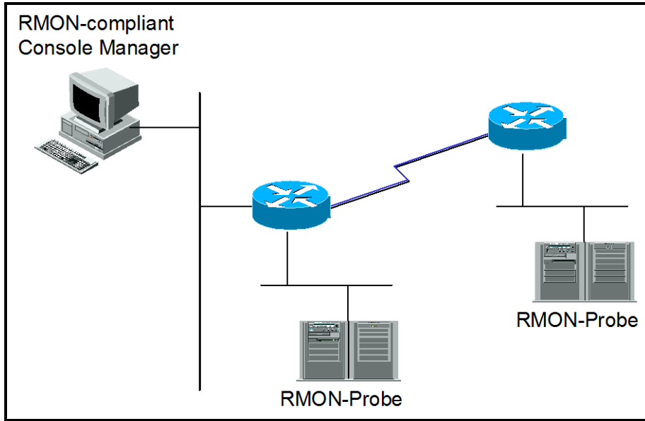
그림 10-1. RMON Manager 와 RMON Probe
