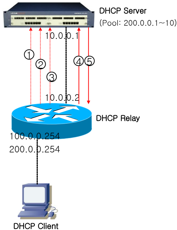
그림 6-3. DHCP Smart-Relay 동작 절차
