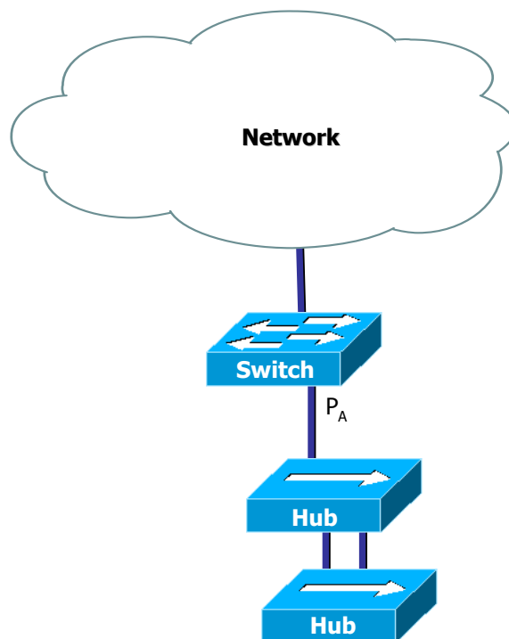
그림 8-4. self-loop 발생 환경
