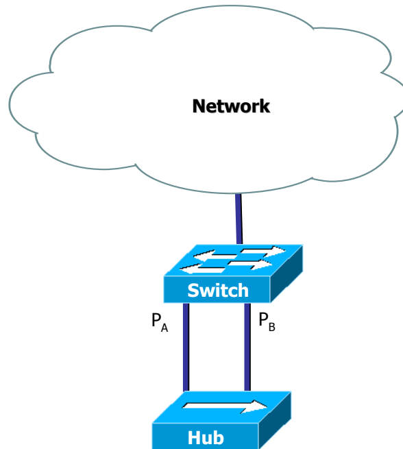
그림 8-5. self-loop 발생 환경 2
