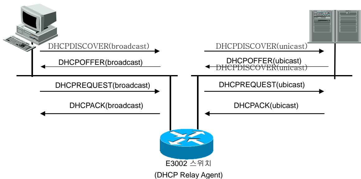
그림 6-1. DHCP Relay Agent 로서 DHCP Server 의 메시지 전달
