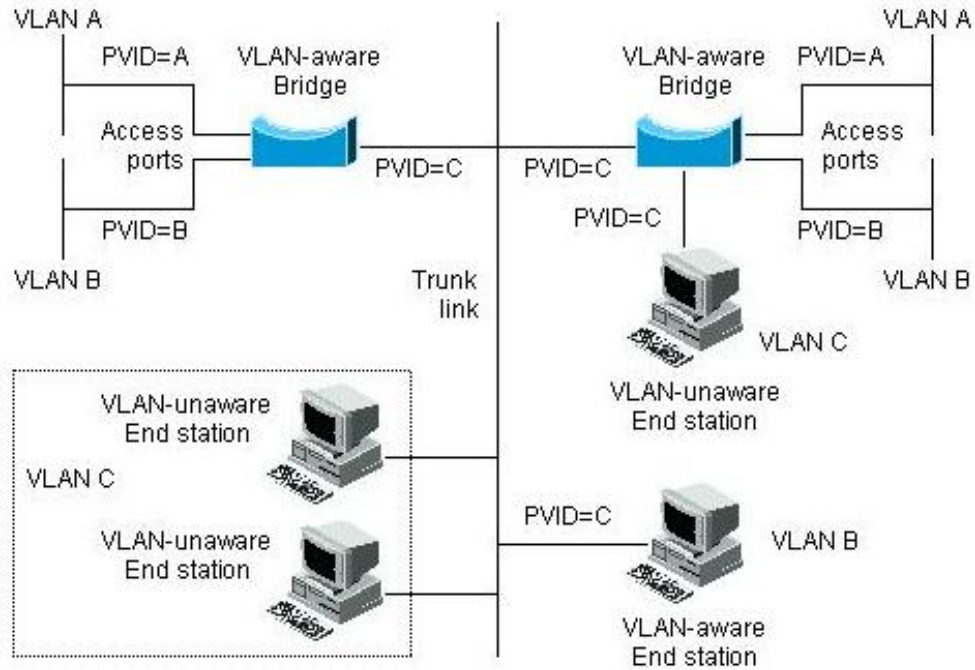
그림 4-6. Native VLAN
