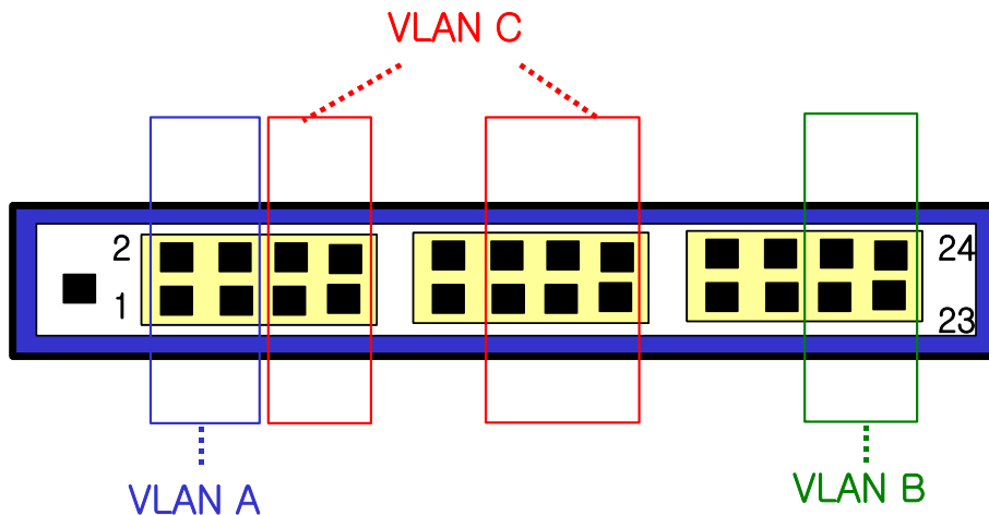
그림 4-1. E3002 Series 스위치의 포트 기반 VLAN 구성 예
