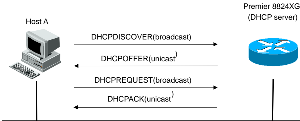
그림 6-1. Premier 8824XG 스위치를 DHCP Server 로 사용
