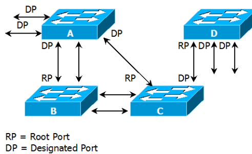
그림 13-1 Spanning-Tree Topology
