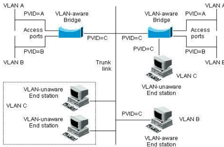
그림 4-6. Native VLAN
