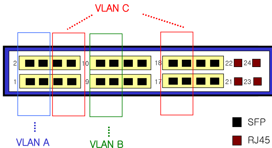
그림 4-1. Premier 8824XG 스위치의 포트 기반 VLAN 구성 예
