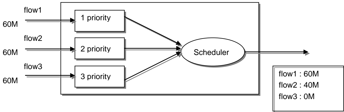
■ 그림 3. SPQ(Strict Priority Queue) Method
