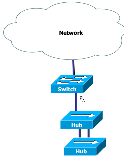
그림 4 self-loop 발생 환경
