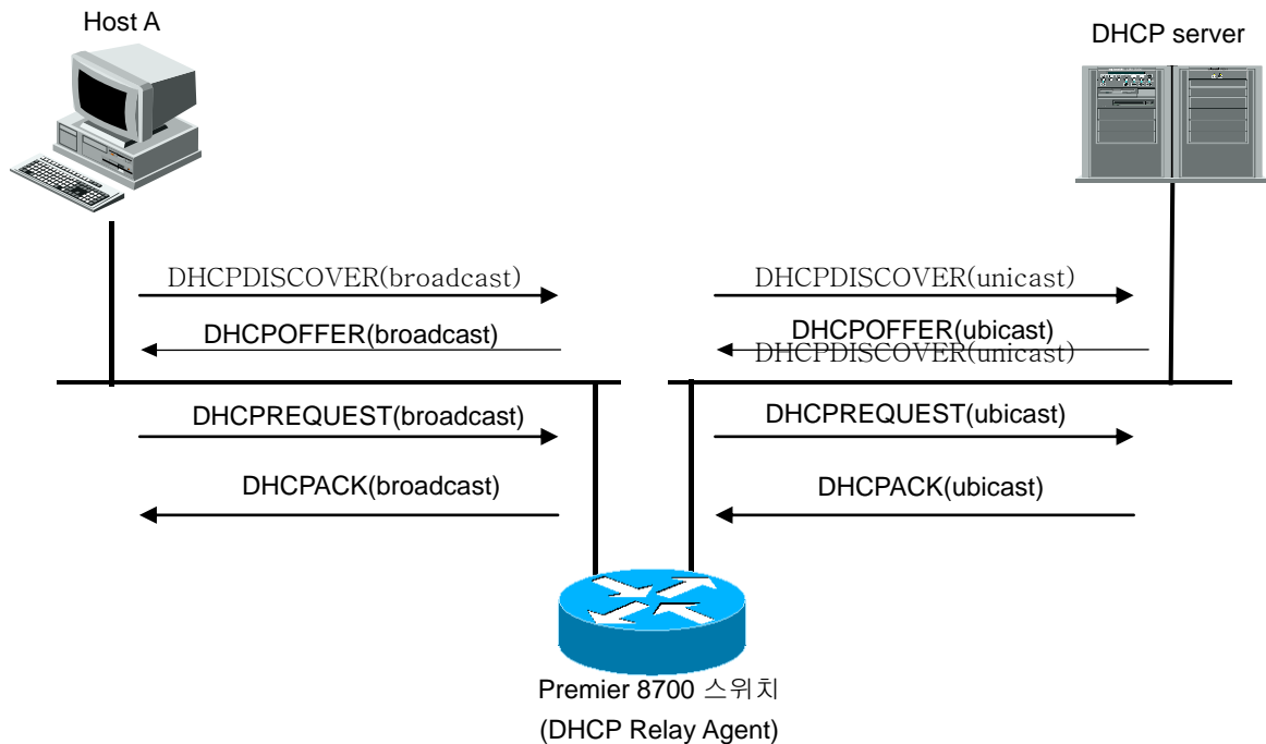
그림 6-3. DHCP Relay Agent 로서 DHCP Server 의 메시지 전달
