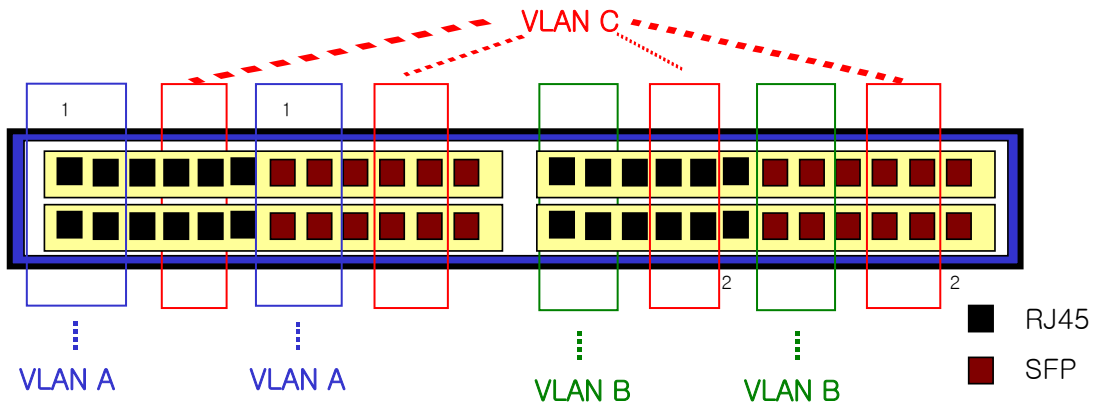
그림 4-1. Premier 8724XG 스위치의 포트 기반 VLAN 구성 예
