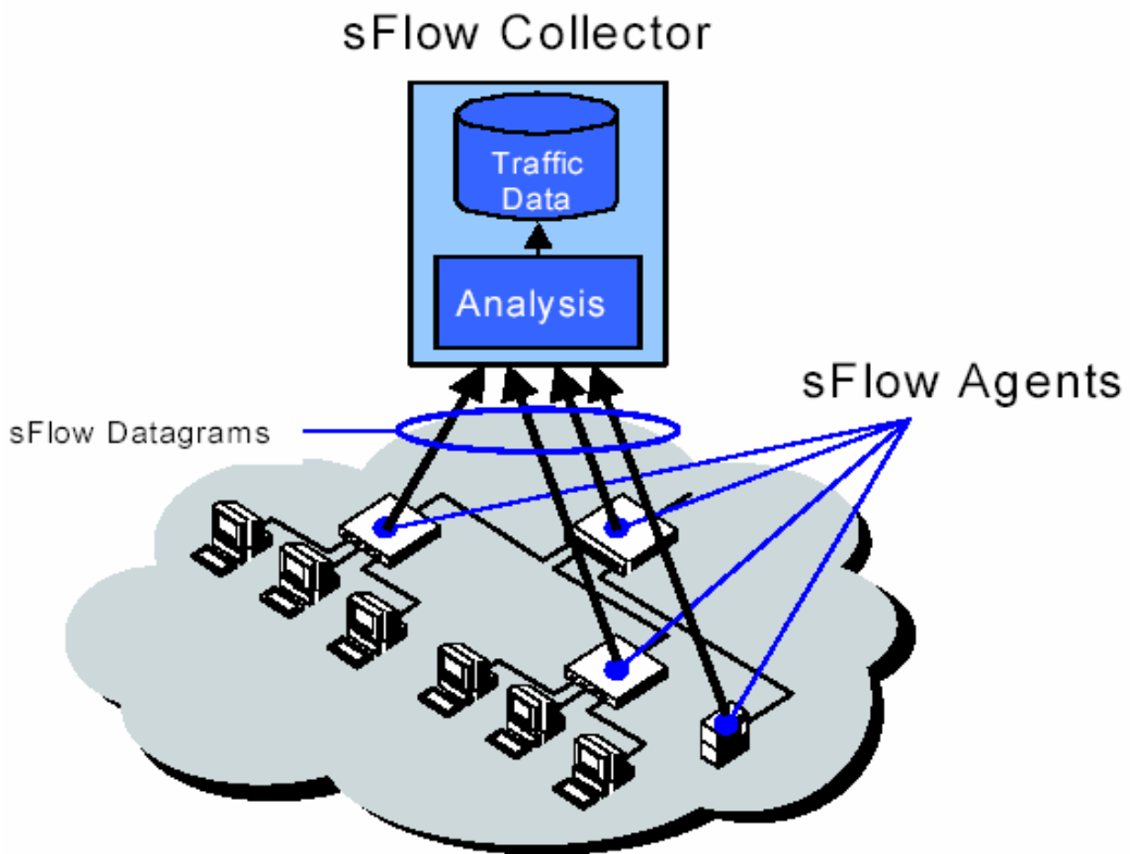
■ 그림 6. sFlow 개념도(sFlow agent 와 collector)
