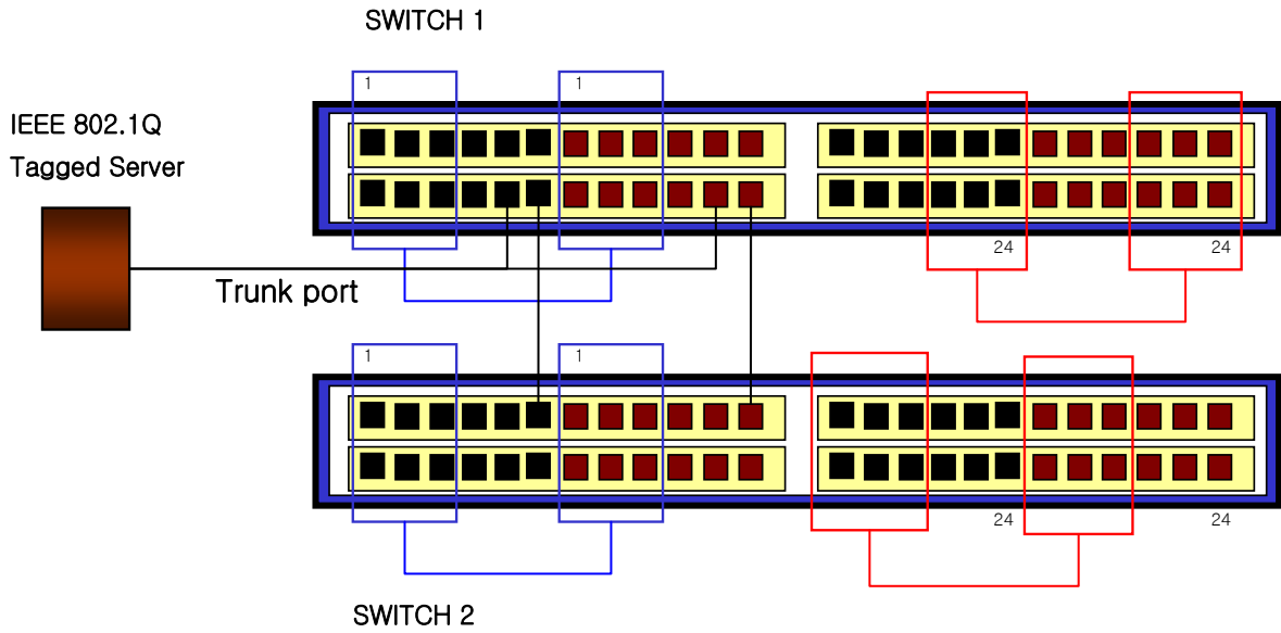
그림 4-4. 태그가 붙은 프레임과 태그가 붙지 않은 프레임의 물리적 다이어그램
