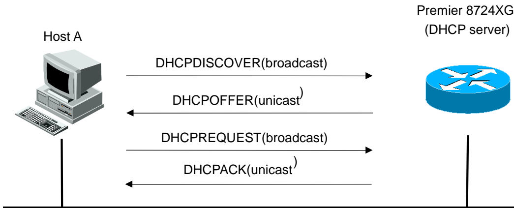
그림 6-1. Premier 8724XG 스위치를 DHCP Server 로 사용
