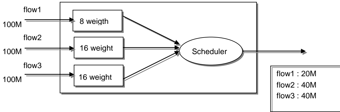
■ 그림 4. WRR(Weighted Round Robin) Method
