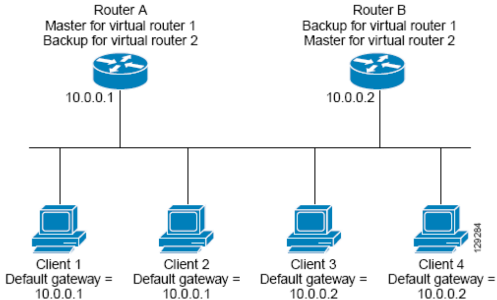
그림 17-2 Load Sharing and Redundancy VRRP Topology
