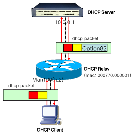
그림 6-3. DHCP Relay Option82
