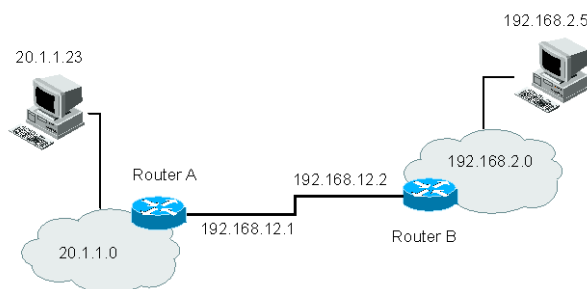
그림 5-2. 네트워크 설정 예 - Static route
