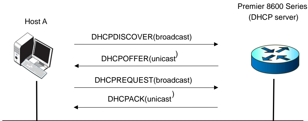
그림 6-1. Premier 8600 Series 스위치를 DHCP Server 로 사용
