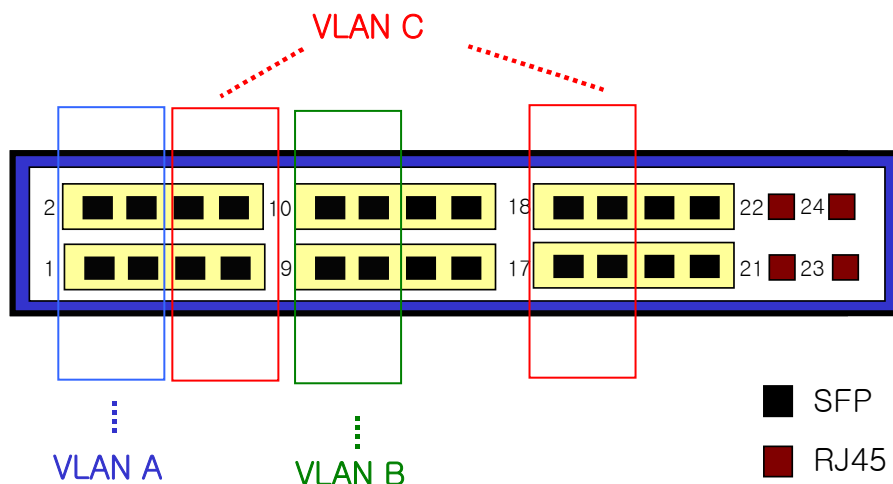
그림 4-1. Premier 8600 Series 스위치의 포트 기반 VLAN 구성 예
