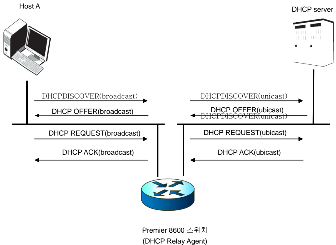
그림 6-2. DHCP Relay Agent 로서 DHCP Server 의 메시지 전달
