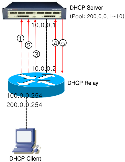
그림 6-3. DHCP Smart-Relay 동작 절차
