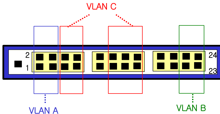
그림 4-1. Premier 3508FG 스위치의 포트 기반 VLAN 구성 예
