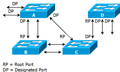
그림 8-1. Spanning-Tree Topology
