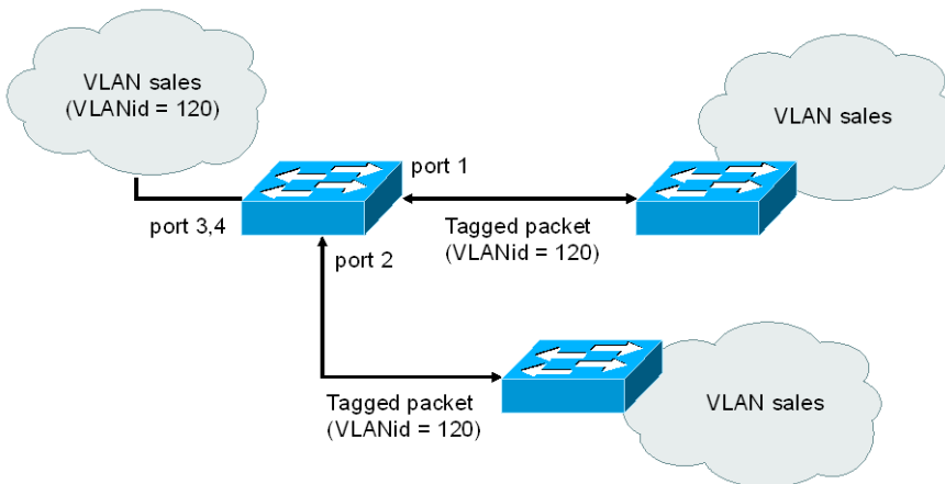
그림 4-7. VLAN 설정 예제 – Tagged and Untagged VLAN
