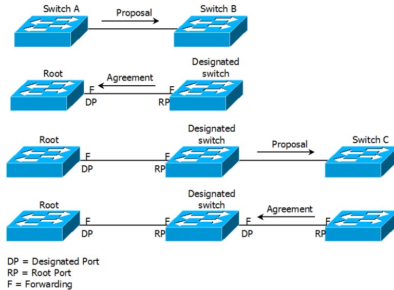
그림 8-2. Proposal and Agreement Handshaking for Rapid Convergence
