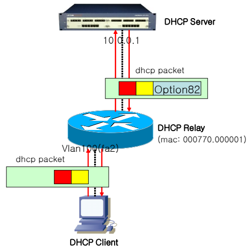
그림 6-2. DHCP Relay Option82
