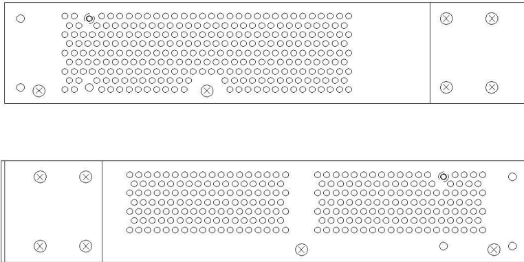
그림 1-13. E5024 좌/우 측면형상
