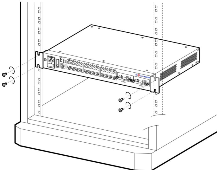
그림 3-1. E5024 랙 설치도
