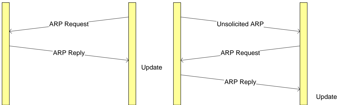
그림 13-1. ARP snoop (3-way handshake)
