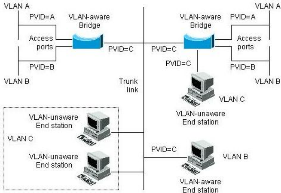
그림 4-6. Native VLAN
