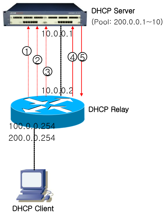
그림 6-3. DHCP Smart-Relay 동작 절차
