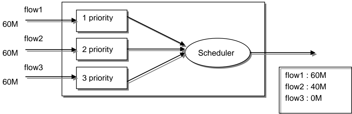
그림 9-2. SPQ(Strict Priority Queue) Method
