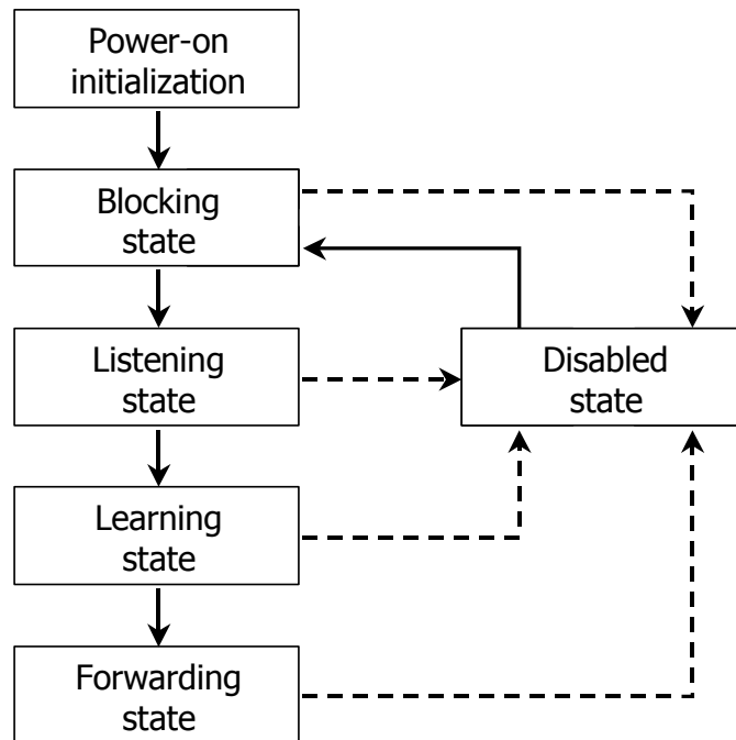
그림 8-2 Spanning-Tree Interface States
