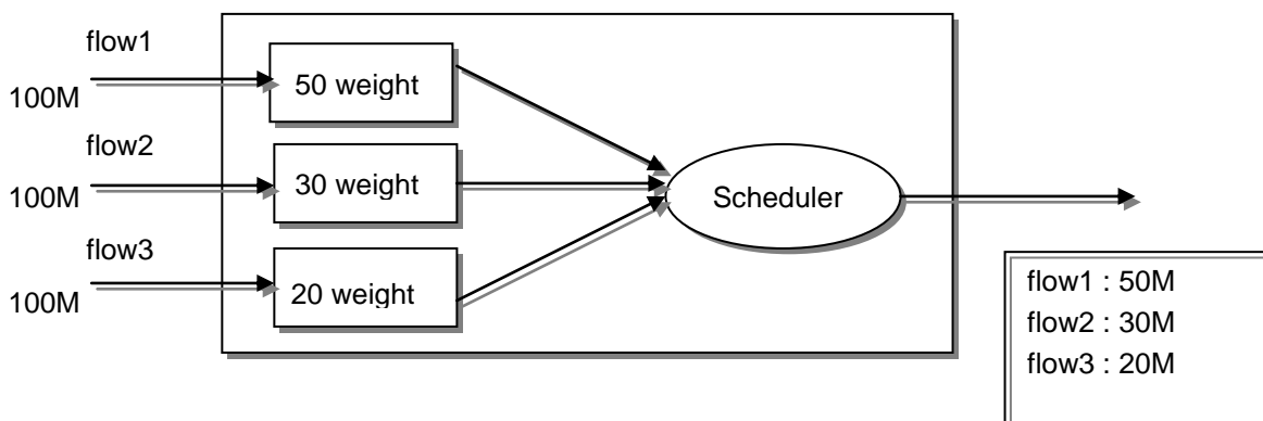
그림 9-3. WRR Method
