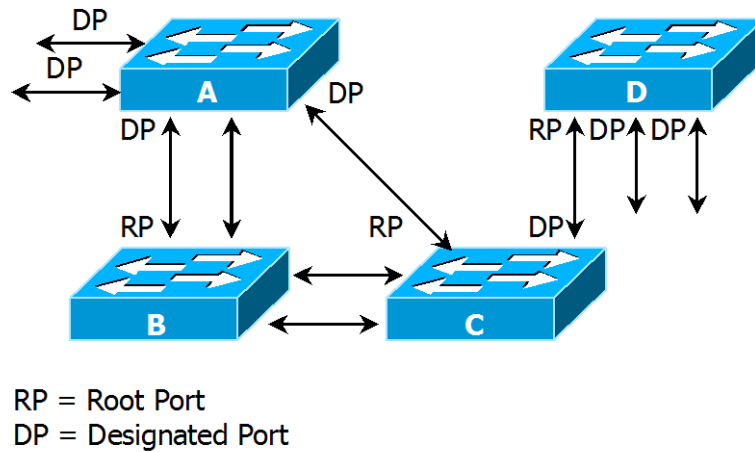
그림 8-1 Spanning-Tree Topology
