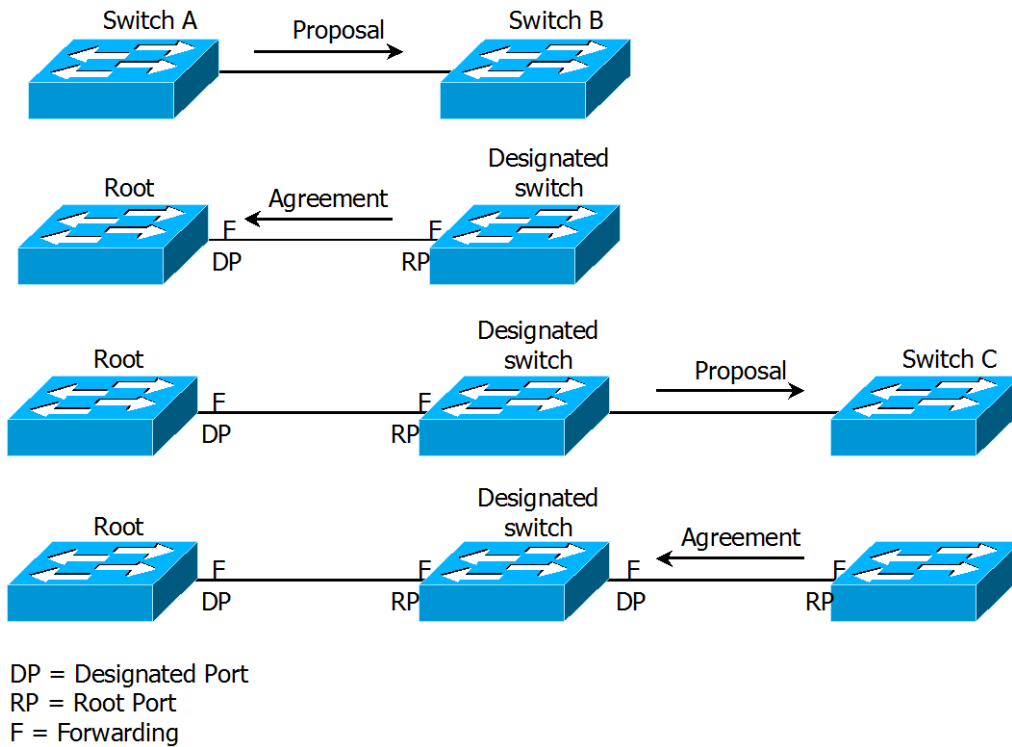
그림 8-3. Proposal and Agreement Handshaking for Rapid Convergence
