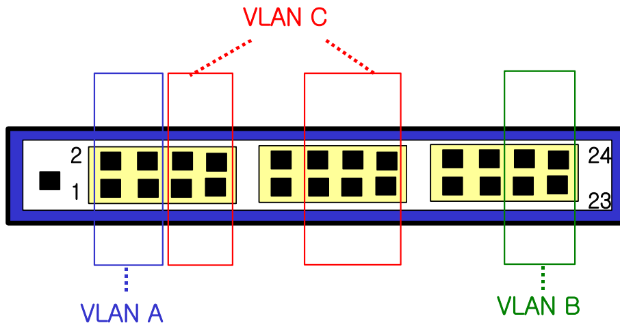
그림 4-1. E50XX Series 스위치의 포트 기반 VLAN 구성 예
