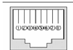
그림6. 콘솔포트 핀 번호
